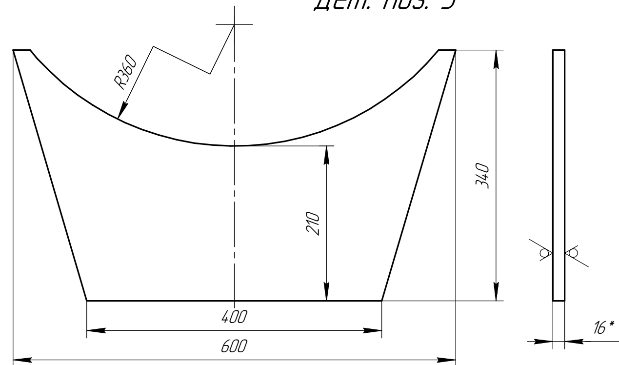
Дет. поз. 3
