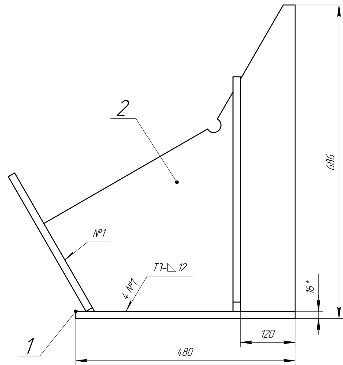
Дет. поз. 1
