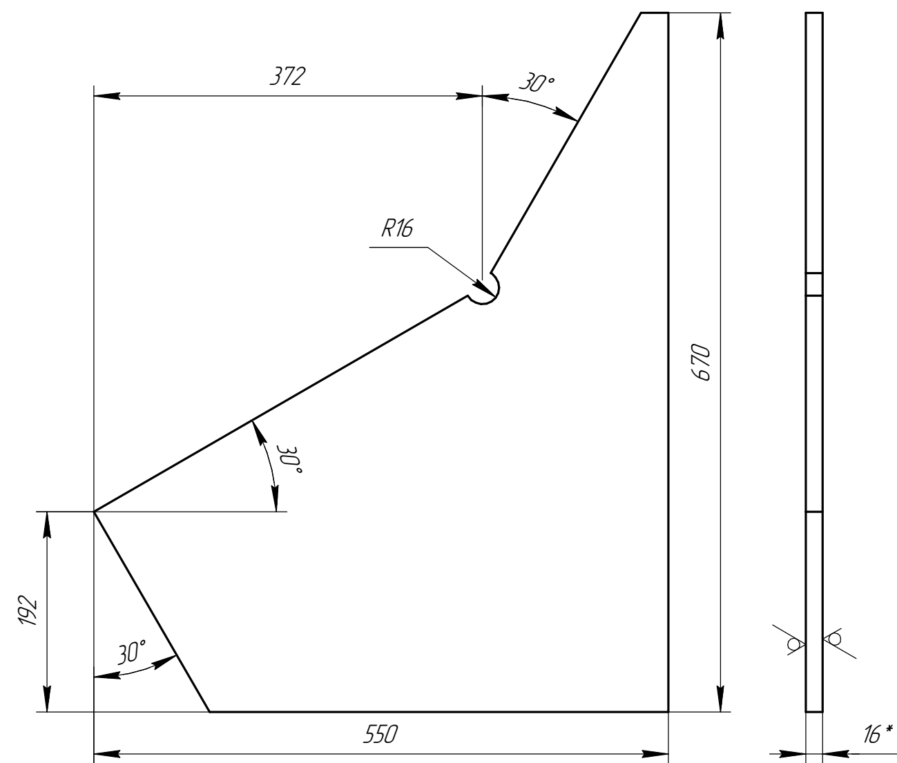
Дет. поз. 2
