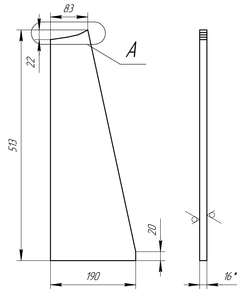
Дет. поз. 4
